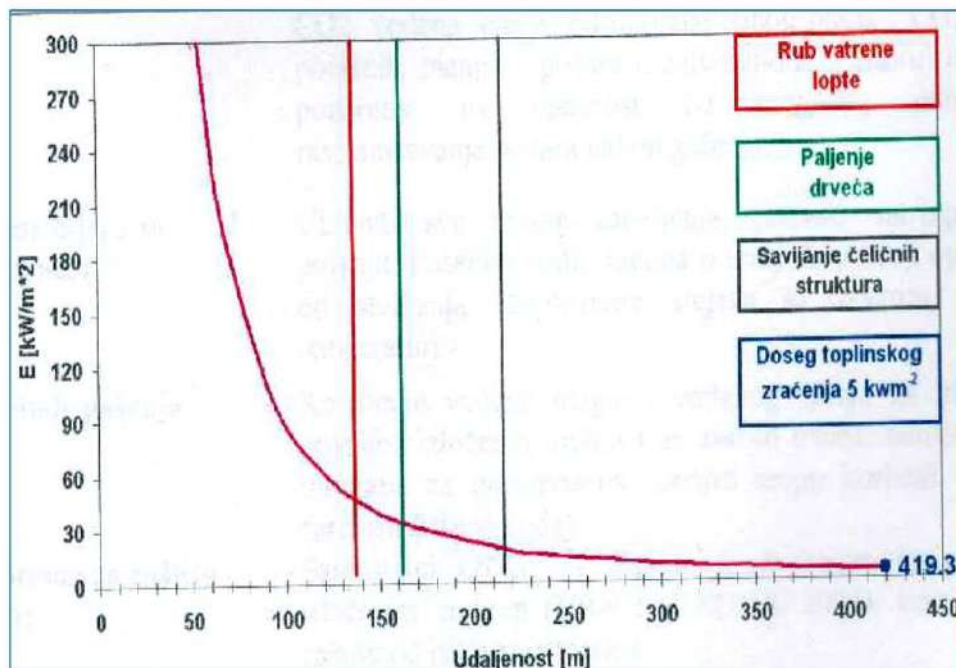
Slika 5.8.-2. – Ovisnost toplinskog toka o udaljenosti od požara
