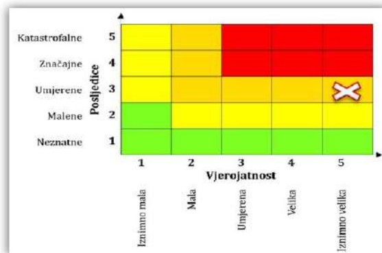
Slika 5.3.-1. - Zbirna matrica rizika u slučaju toplinskih valova na području Općine Stari Jankovci
