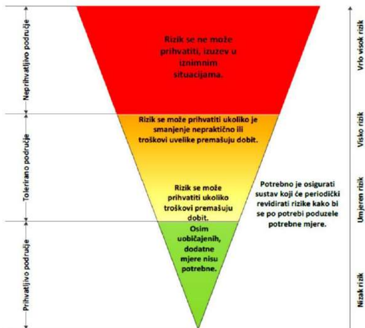
Slika 8. - 1. Vrednovanje rizika - ALARP načela
